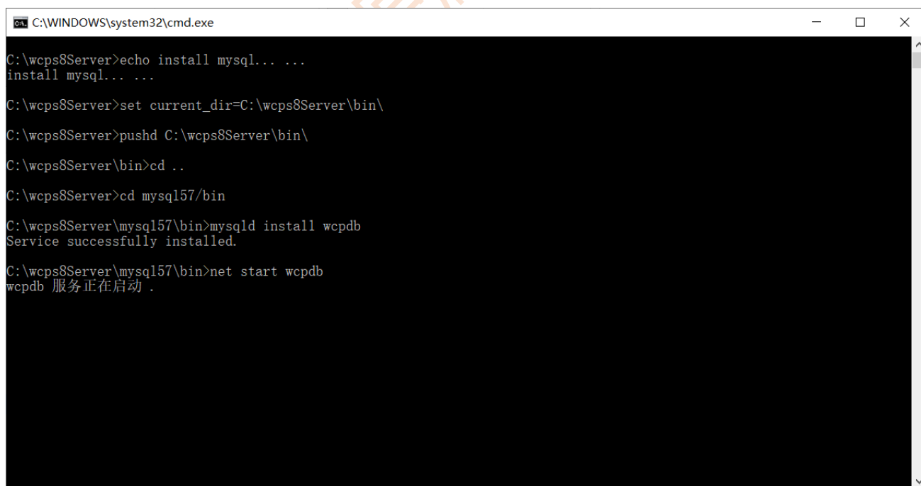
上图：等待数据库服务安装
